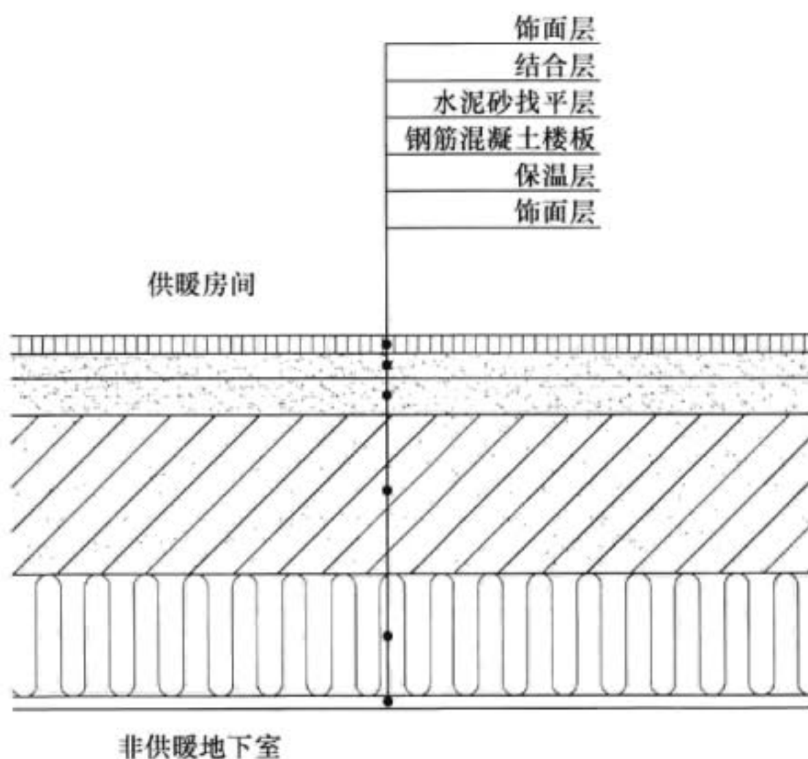
图 11 非供暖地下室顶板保温构造做法 2
