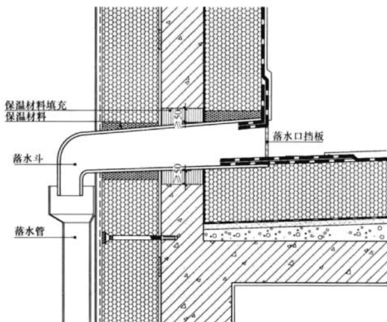
图 9 落水管处做法
