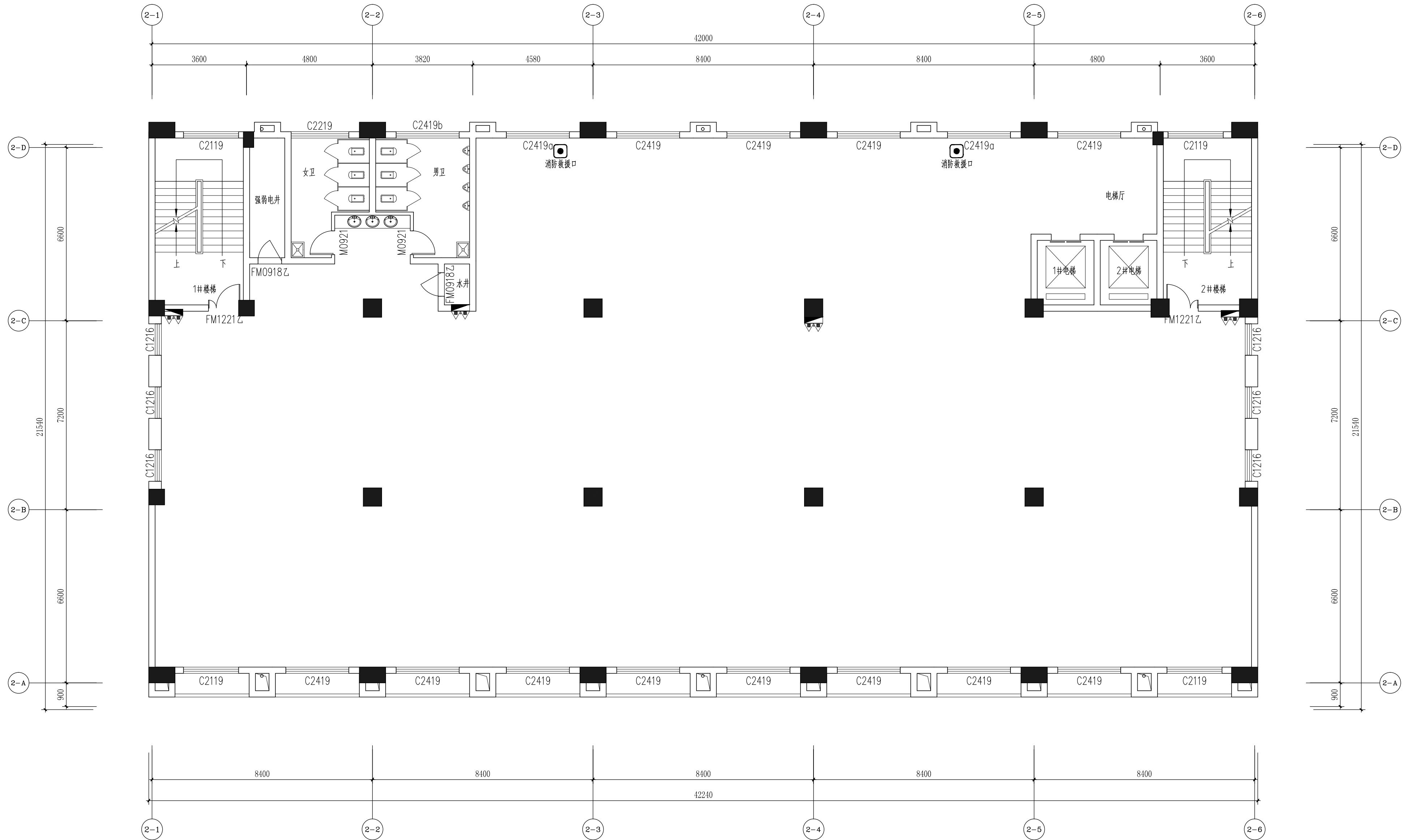
四层原始结构图 比例1: 100
