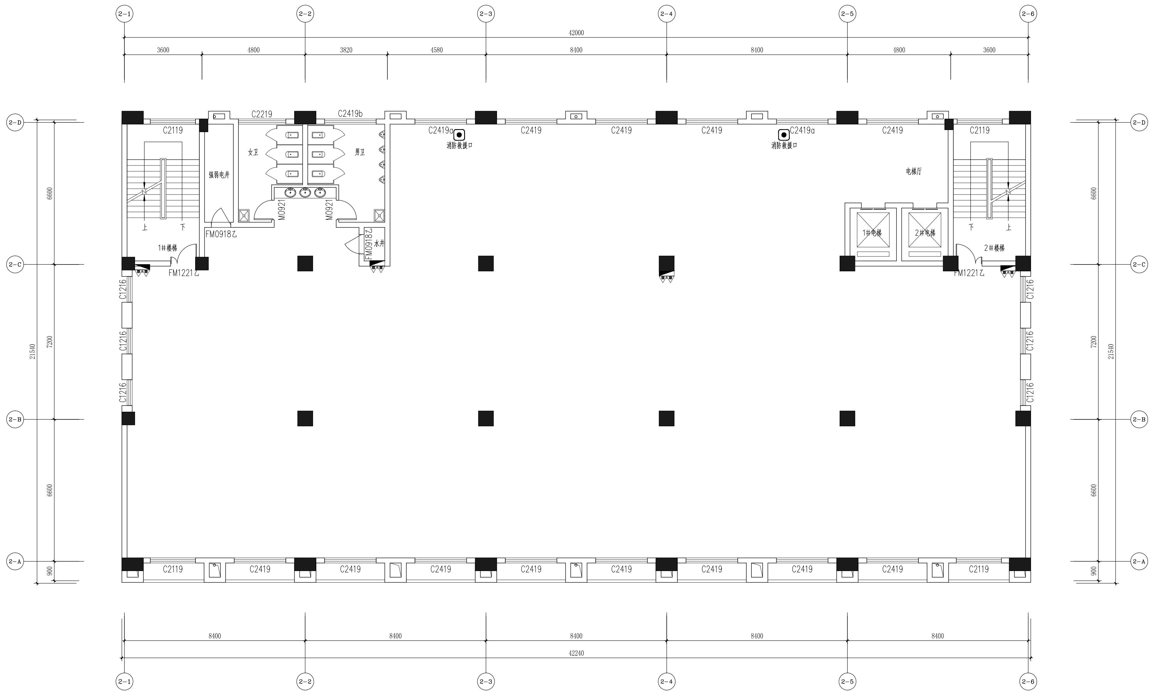
六层原始结构图 比例1: 100
