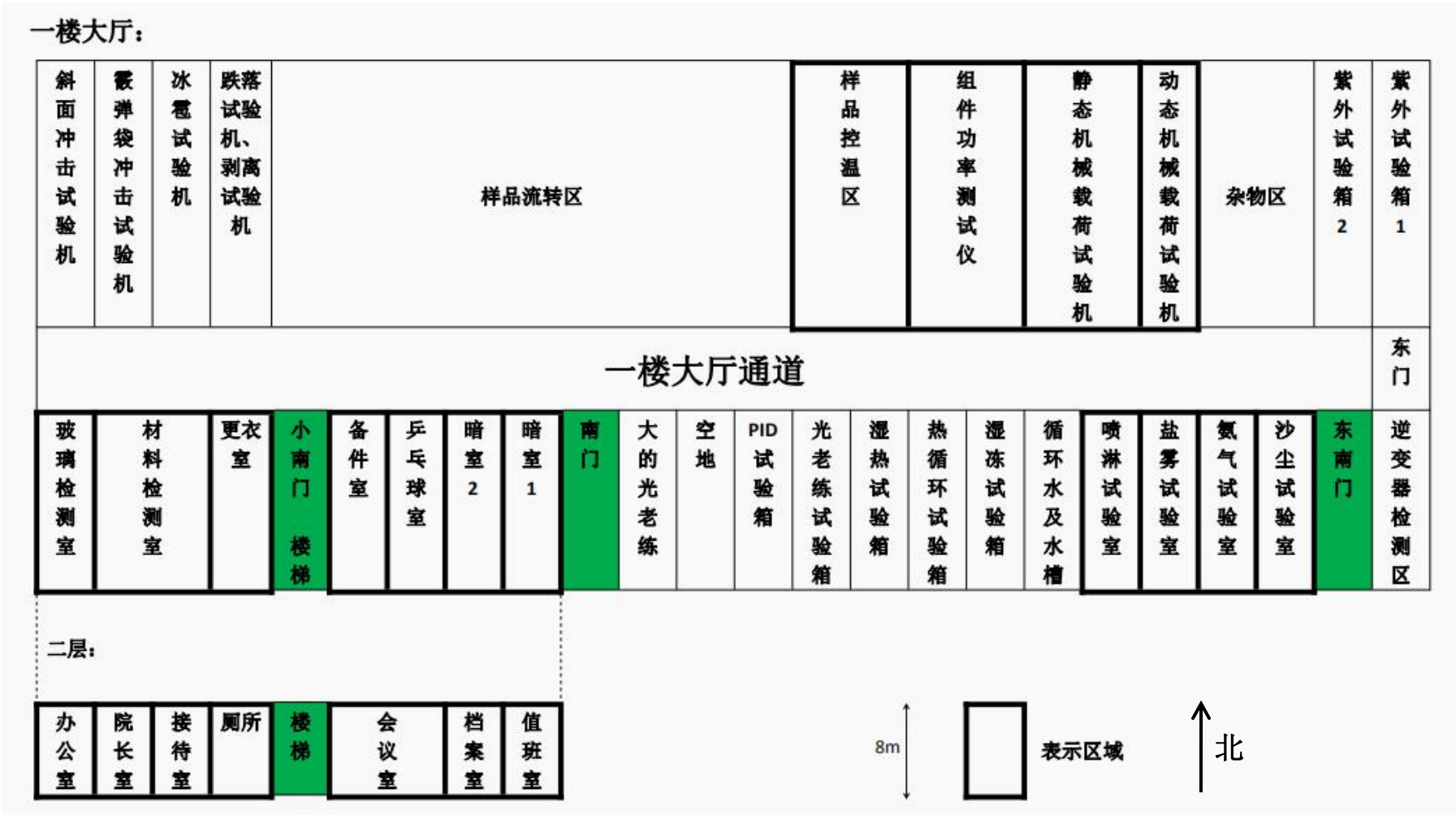
附图 3-2：光伏实验室平面布置图
